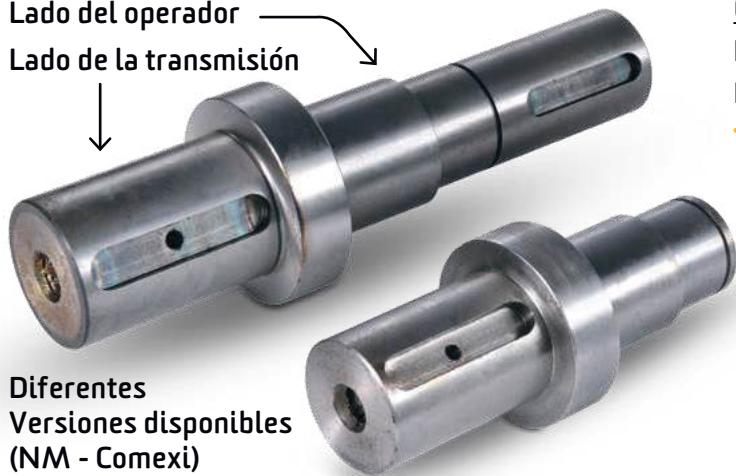
Eje para cono dentado
